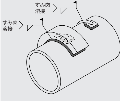
図1：溶接模式図
