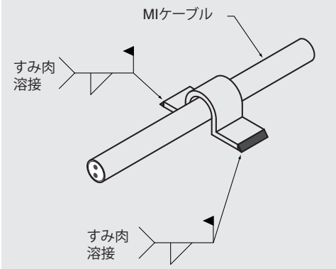
図2：チューブクリップ溶接模式図
