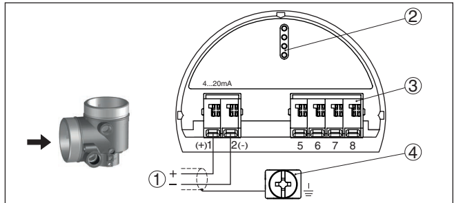
Abb. 32: Anschlussraum - Zweikammergehäuse
