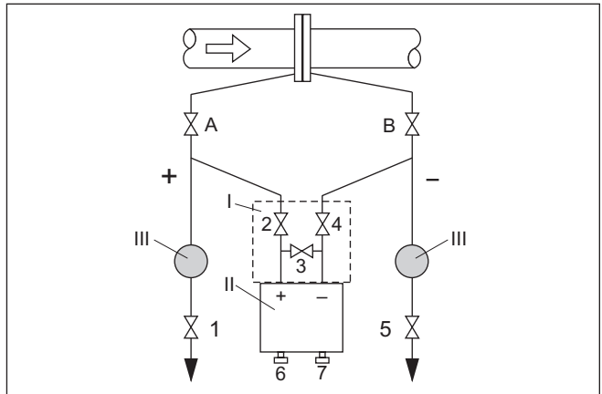
Abb. 46: Bevorzugte Messanordnung für Flüssigkeiten
