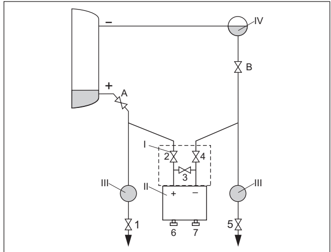
Abb. 44: Bevorzugte Messanordnung für geschlossene Behälter mit Dampfüberlagerung
