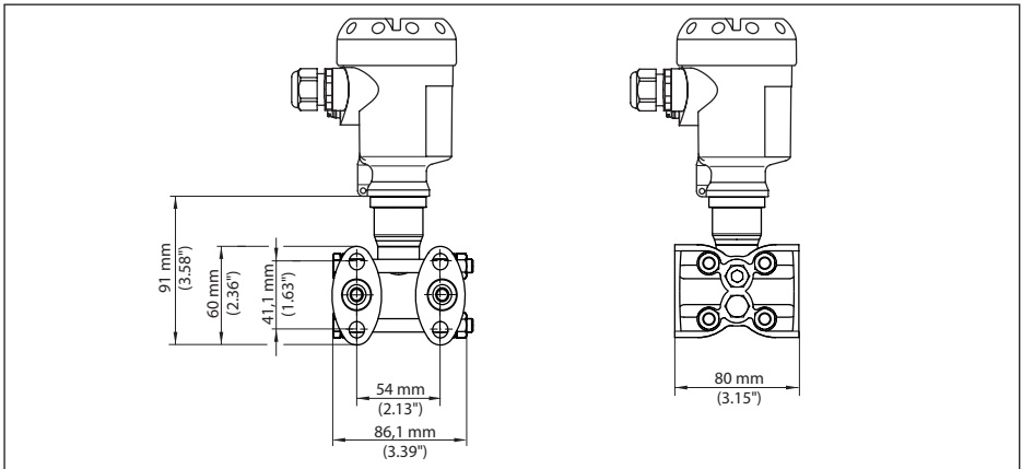
Abb. 53: DPT-20, Entlüftung seitlich
