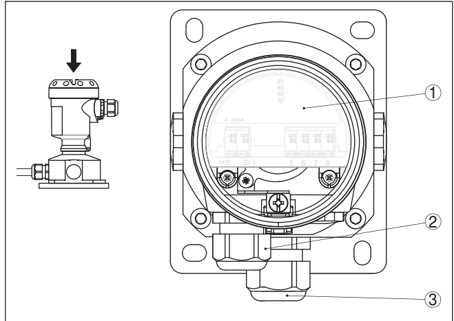
Abb. 34: Elektronik- und Anschlussraum
