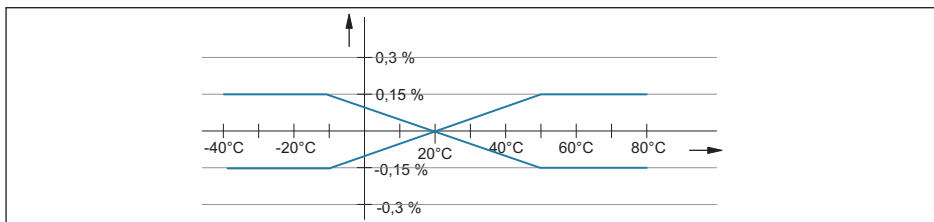
Abb. 50: Thermische Änderung Stromausgang
