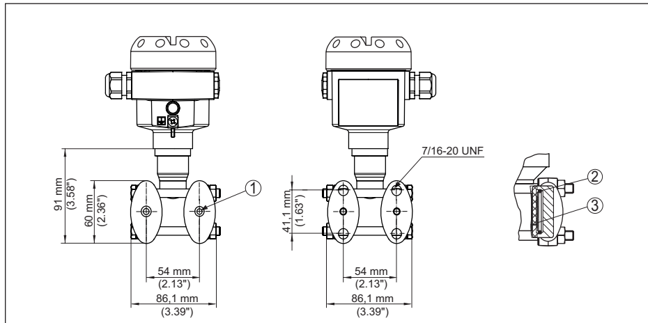
Abb. 54: links: Prozessanschluss DPT-20 vorbereitet für den Druckmittlerbau. Rechts: Lage der Kupferingdichtung
