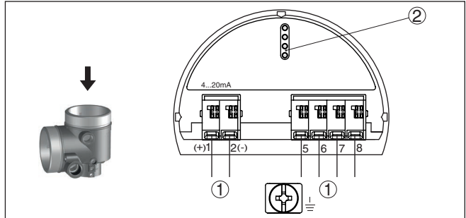
Abb. 31: Elektronikraum - Ex-d-Zweikammergehäuse
