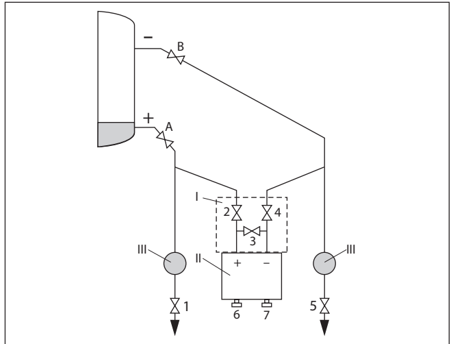
Abb. 43: Bevorzugte Messanordnung für geschlossene Behälter
