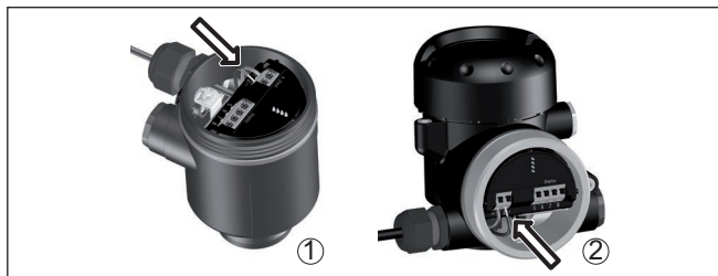
Abb. 26: Anschlusschritte 5 und 6
