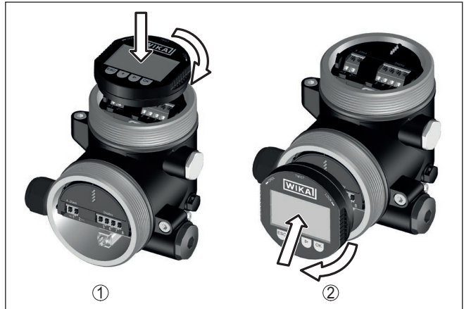
Abb. 39: Einsetzen des Anzeige- und Bedienmoduls beim Zweikammergehäuse
