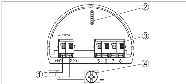
Abb. 36: Elektronik- und Anschlussraum - Einkammergehäuse
