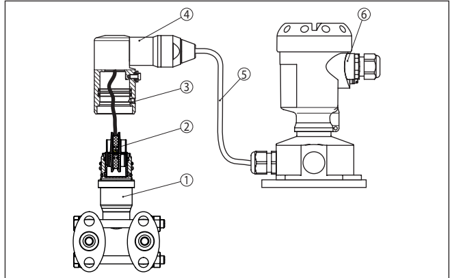
Abb. 48: DPT-20 in IP68-Ausführung 25 bar und seitlichem Kabelabgang, externes Gehäuse
