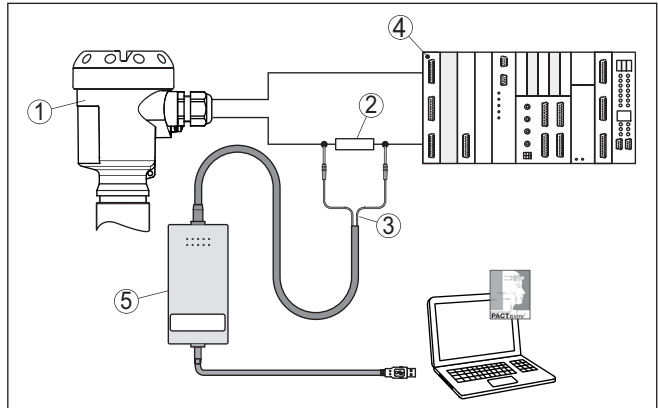
Abb. 42: Anschluss des PCs via HART an die Signalleitung
