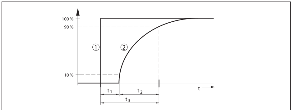
Abb. 49: Verhalten bei sprunghafter Änderung der Prozessgröße. t_1 : Totzeit; t_2 : Anstiegszeit; t_3 : Sprungantwortzeit
