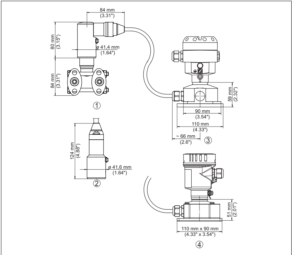
Abb. 51: Externes Gehäuse
