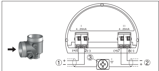
Abb. 30: Anschlussraum Zweikammergehäuse, Zusatzelektronik "Zusätzlicher Stromausgang"
