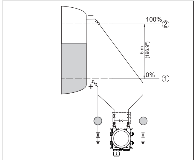
Abb. 41: Parametrierbeispiel Min.-/Max.-Abgleich Füllstandmessung
