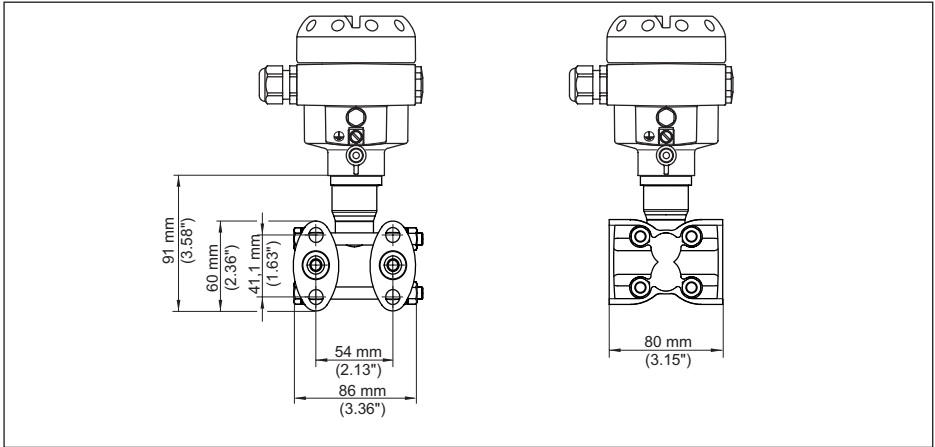
Abb. 52: DPT-20, Entlüftung auf Prozessachse
