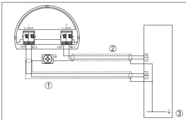
Abb. 37: Anschlussbeispiel DPT-20 zusätzlicher Stromausgang
