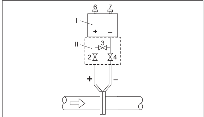
Abb. 45: Bevorzugte Messanordnung für Gase, Anschluss über 3-fach-Ventilblock, beidseitig anflanschbar
